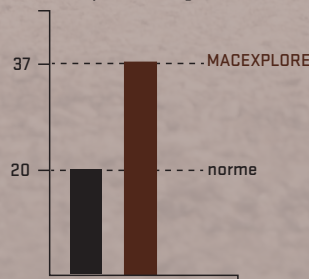
Absorption d'énergie en Joule [J]
